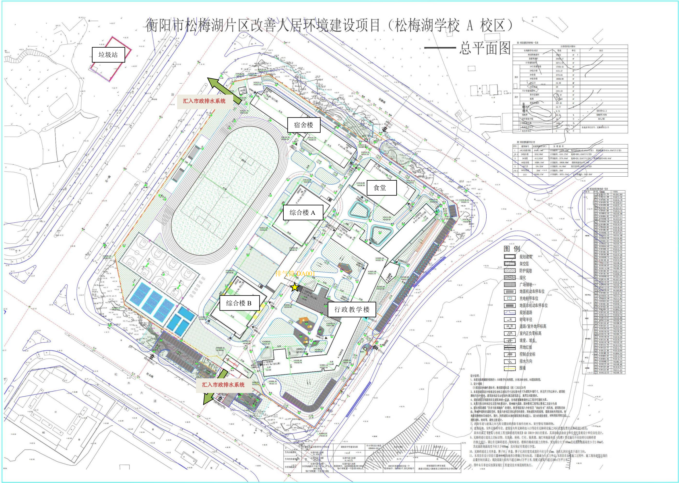
附图 2 总平面布置图
